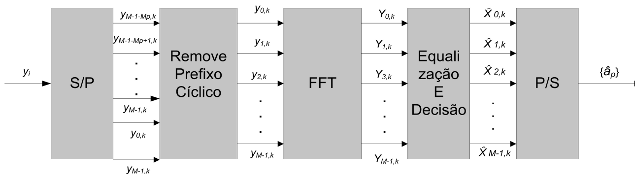
Figura 2. Diagrama de blocos do receptor OFDM
