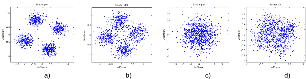
Figura 4. Scatterplot : (a) Portadora 1 com o canal dispersivo no tempo não-equalizado (b) Portadora 3 com o canal dispersivo no tempo não-equalizado (c) Portadora 5 com o canal dispersivo no tempo não-equalizado (d) Portadora 7 com o canal dispersivo no tempo não-equalizado
