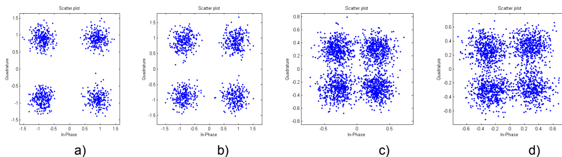
Figura 5. Scatterplot: (a) Portadora 1 equalizada (b) Portadora 3 equalizada (c) Portadora 5 equalizada (d) Portadora 7 equalizada
